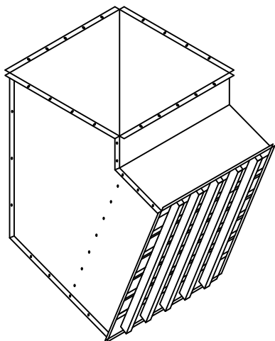
45° DIFFUSER
